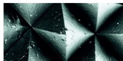
Wzór materiału ściernego 3M™ Trizact™ widoczny pod mikroskopem
